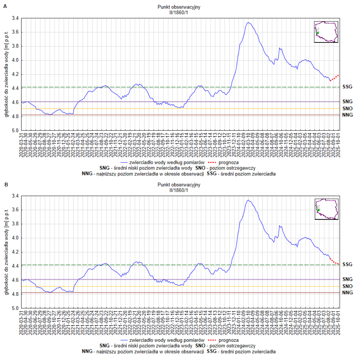
Rys. 7. Prognoza dotycząca stanu wód o zwierciadle swobodnym (gruntowych) na okres 01.09.2025 –30.09.2025 r. – stacja hydrogeologiczna nr II/1860/1 w miejscowości Szprotawa (woj. lubuskie) A – prognoza przy założeniu scenariusza A; B – prognoza przy założeniu scenariusza B
