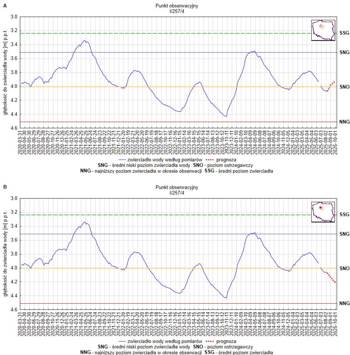
Rys. 4. Prognoza dotycząca stanu wód o zwierciadle swobodnym (gruntowych) na okres 01.09.2025 – 30.09.2025 r. – stacja hydrogeologiczna nr I/257/4 w miejscowości Jagodowo (woj. kujawsko-pomorskie). A – prognoza przy założeniu scenariusza A; B – prognoza przy założeniu scenariusza B
