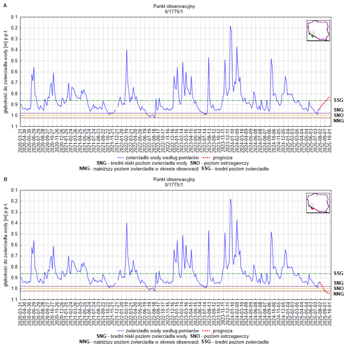
Rys. 2. Prognoza dotycząca stanu wód o zwierciadle swobodnym (gruntowych) na okres 01.09.2025 –30.09.2025 r. – stacja hydrogeologiczna nr II/1775/1 w miejscowości Różanka (woj. dolnośląskie). A – prognoza przy założeniu scenariusza A; B – prognoza przy założeniu scenariusza B
