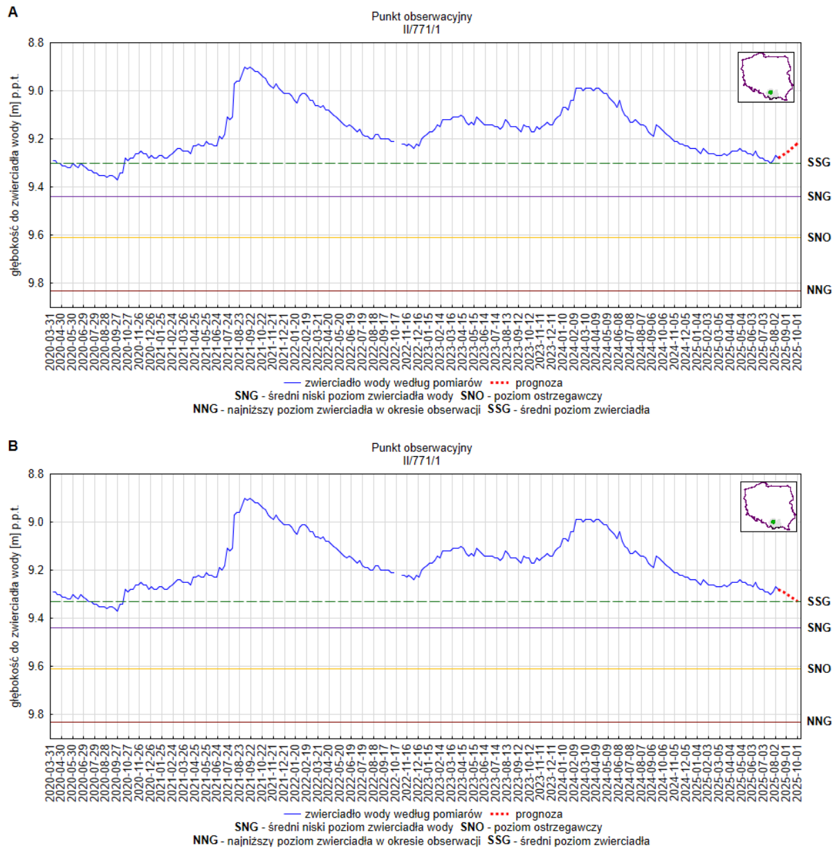
Rys. 11. Prognoza dotycząca stanu wód o zwierciadle swobodnym (gruntowych) na okres 01.09.2025 –30.09.2025 r. – stacja hydrogeologiczna nr II/771/1 w miejscowości Kraków (woj. małopolskie). A – prognoza przy założeniu scenariusza A; B – prognoza przy założeniu scenariusza B
