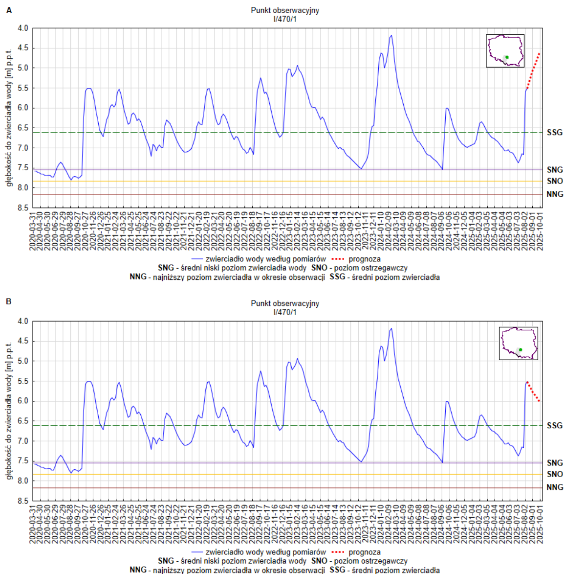
Rys. 19. Prognoza dotycząca stanu wód o zwierciadle swobodnym (gruntowych) na okres 01.09.2025 – 30.09.2025 r. – stacja hydrogeologiczna nr I/470/1 w miejscowości Podlesie (woj. śląskie). A – prognoza przy założeniu scenariusza A; B – prognoza przy założeniu scenariusza B
