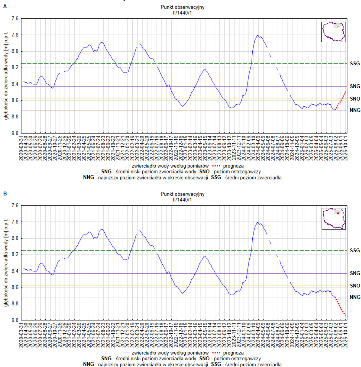
Rys. 21. Prognoza dotycząca stanu wód o zwierciadle swobodnym (gruntowych) na okres 01.09.2025 –30.09.2025 r. – stacja hydrogeologiczna nr II/1440/1 w miejscowości Zieleniec (woj. warmińsko-mazurskie). A – prognoza przy założeniu scenariusza A; B – prognoza przy założeniu scenariusza B
