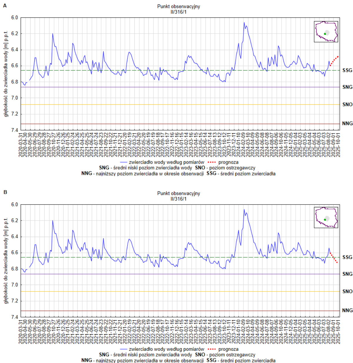
Rys. 9. Prognoza dotycząca stanu wód o zwierciadle swobodnym (gruntowych) na okres 01.09.2025 –30.09.2025 r. – stacja hydrogeologiczna nr II/316/1 w miejscowości Masłowice (woj. łódzkie). A – prognoza przy założeniu scenariusza A; B – prognoza przy założeniu scenariusza B
