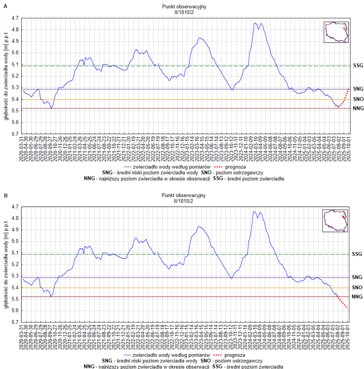
Rys. 16. Prognoza dotycząca stanu wód o zwierciadle swobodnym (gruntowych) na okres 01.09.2025 –30.09.2025 r.- stacja hydrogeologiczna nr II/1810/2 w miejscowości Liza Stara (woj. podlaskie). A – prognoza przy założeniu scenariusza A; B – prognoza przy założeniu scenariusza B
