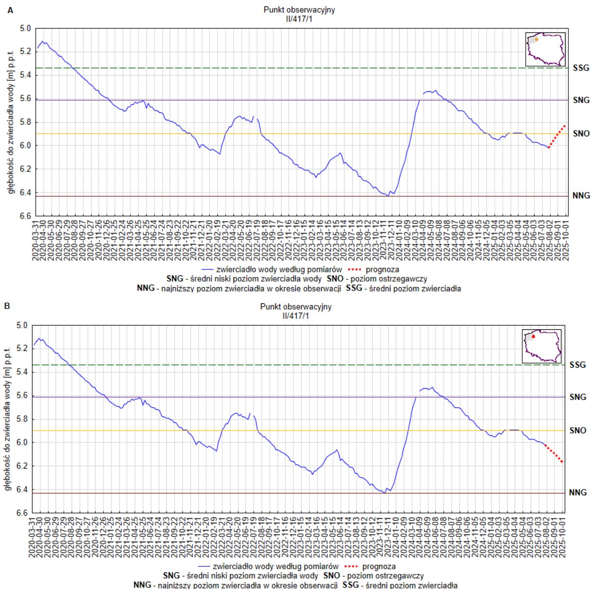
Rys. 25. Prognoza dotycząca stanu wód o zwierciadle swobodnym (gruntowych) na okres 01.09.2025 –30.09.2025 r. – stacja hydrogeologiczna nr II/417/1 w miejscowości Turowo (woj. zachodniopomorskie). A – prognoza przy założeniu scenariusza A; B – prognoza przy założeniu scenariusza B
