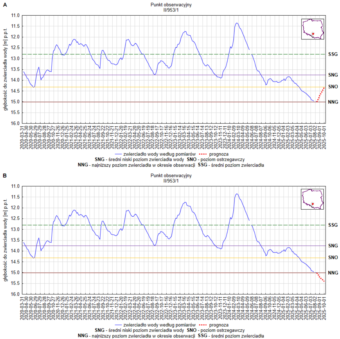
Rys. 18 Prognoza dotycząca stanu wód o zwierciadle swobodnym (gruntowych) na okres 01.09.2025 –30.09.2025 r. – stacja hydrogeologiczna nr II/953/1 w miejscowości Żeliszawice (woj. śląskie). A – prognoza przy założeniu scenariusza A; B – prognoza przy założeniu scenariusza B
