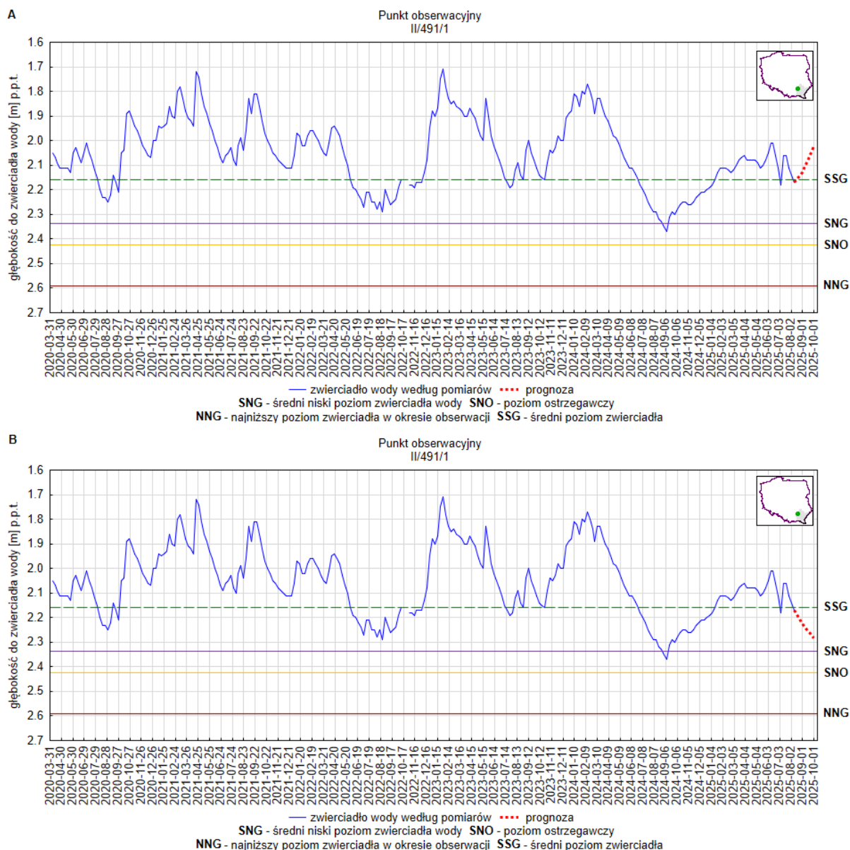
Rys. 15. Prognoza dotycząca stanu wód o zwierciadle swobodnym (gruntowych) na okres 01.09.2025 – 30.09.2025 r. – stacja hydrogeologiczna nr II/491/I w miejscowości Mielec (woj. podkarpackie). A – prognoza przy założeniu scenariusza A; B – prognoza przy założeniu scenariusza B
