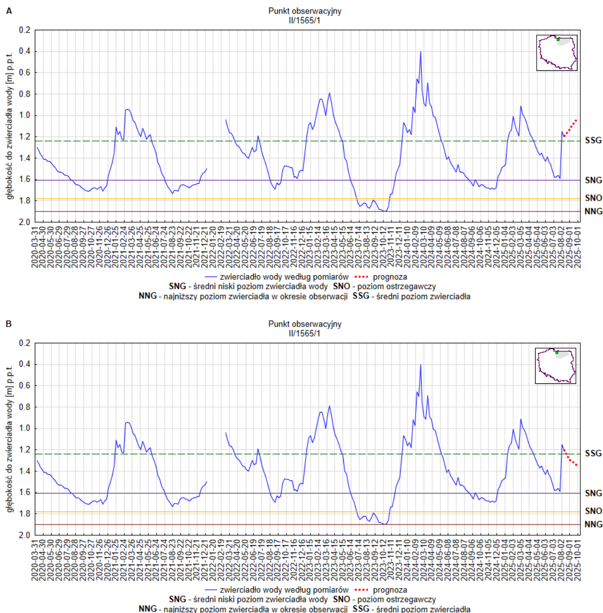
Rys. 22. Prognoza dotycząca stanu wód o zwierciadle swobodnym (gruntowych) na okres 01.09.2025 –30.09.2025 r. – stacja hydrogeologiczna nr II/1565/1 w miejscowości Karczowiska Górne (woj. warmińsko-mazurskie). A – prognoza przy założeniu scenariusza A; B – prognoza przy założeniu scenariusza B
