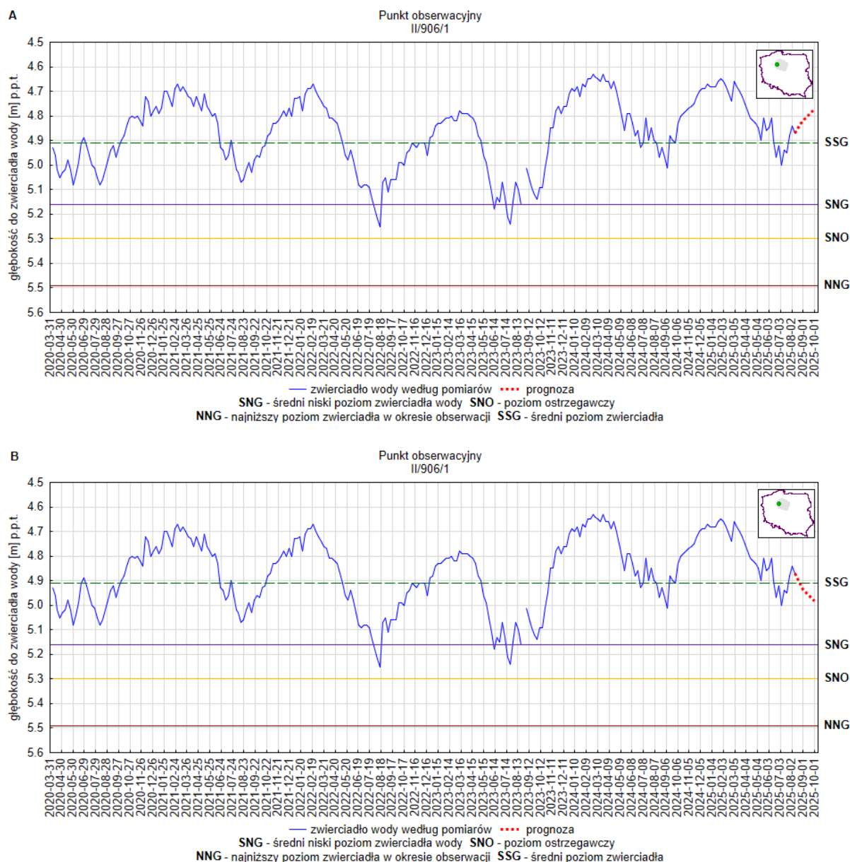
Rys. 5. Prognoza dotycząca stanu wód o zwierciadle swobodnym (gruntowych) na okres 01.09.2025 –30.09.2025 r. – stacja hydrogeologiczna nr II/906/1 w miejscowości Rozwarzyn (woj. kujawsko-pomorskie). A – prognoza przy założeniu scenariusza A; B – prognoza przy założeniu scenariusza B
