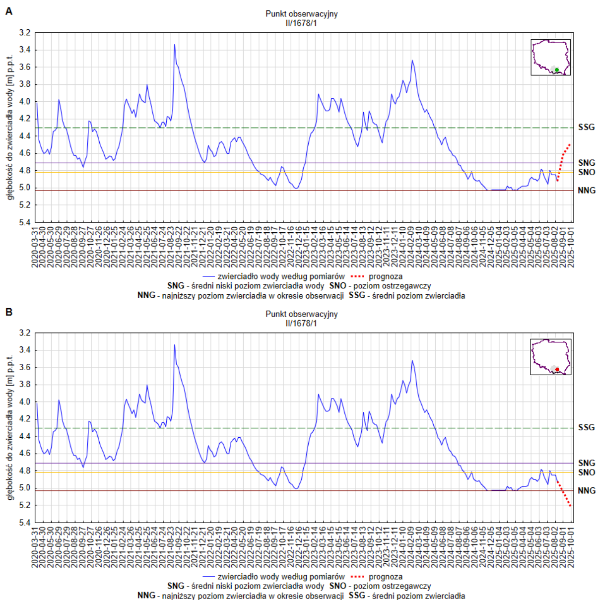
Rys. 10. Prognoza dotycząca stanu wód o zwierciadle swobodnym (gruntowych) na okres 01.09.2025 –30.09.2025 r. – stacja hydrogeologiczna nr II/1678/1 w miejscowości Zakliczyn (woj. małopolskie). A – prognoza przy założeniu scenariusza A; B – prognoza przy założeniu scenariusza B
