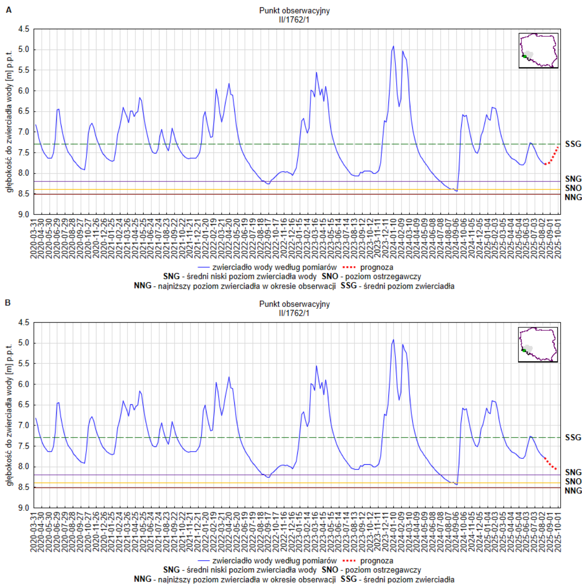
Rys. 3. Prognoza dotycząca stanu wód o zwierciadle swobodnym (gruntowych) na okres 01.09.2025 –30.09.2025 r. – stacja hydrogeologiczna nr II/1762/1 w miejscowości Szklarska Poręba (woj. dolnośląskie). A – prognoza przy założeniu scenariusza A; B – prognoza przy założeniu scenariusza B
