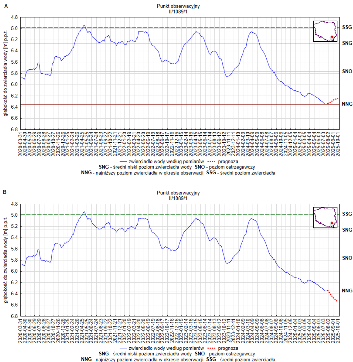
Rys. 14. Prognoza dotycząca stanu wód o zwierciadle swobodnym (gruntowych) na okres 01.09.2025 – 30.09.2025 r. – stacja hydrogeologiczna nr II/1089/1 w miejscowości Turza (woj. podkarpackie). A – prognoza przy założeniu scenariusza A; B – prognoza przy założeniu scenariusza B
