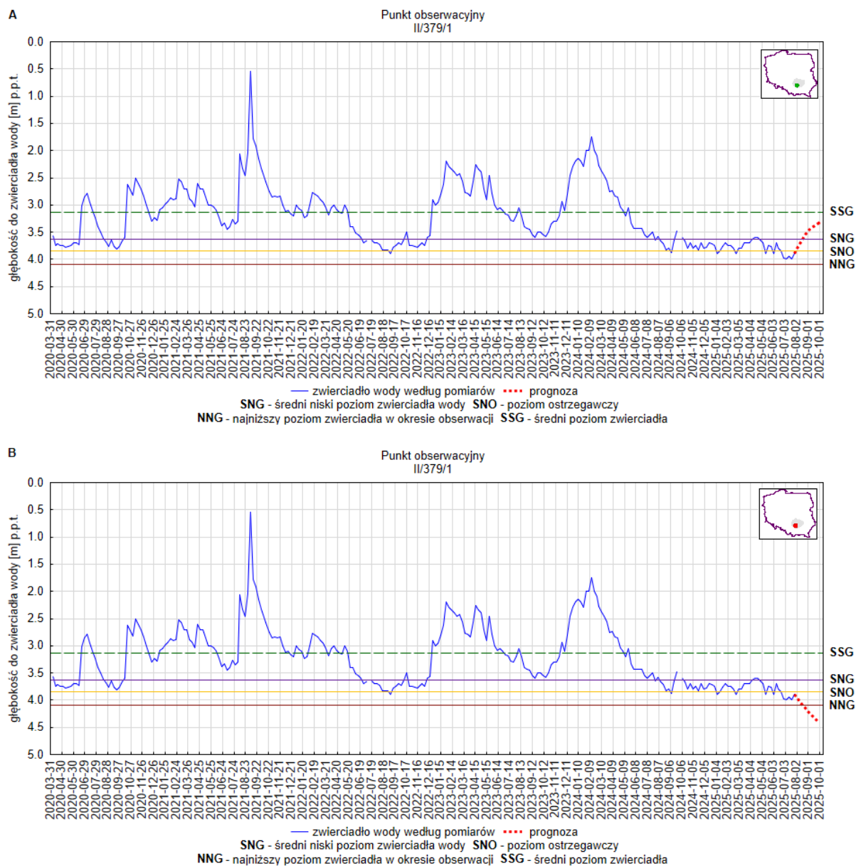
Rys. 20. Prognoza dotycząca stanu wód o zwierciadle swobodnym (gruntowych) na okres 01.09.2025 – 30.09.2025 r. – stacja hydrogeologiczna nr II/379/1 w miejscowości Michałów (woj. świętokrzyskie). A – prognoza przy założeniu scenariusza A; B – prognoza przy założeniu scenariusza B
