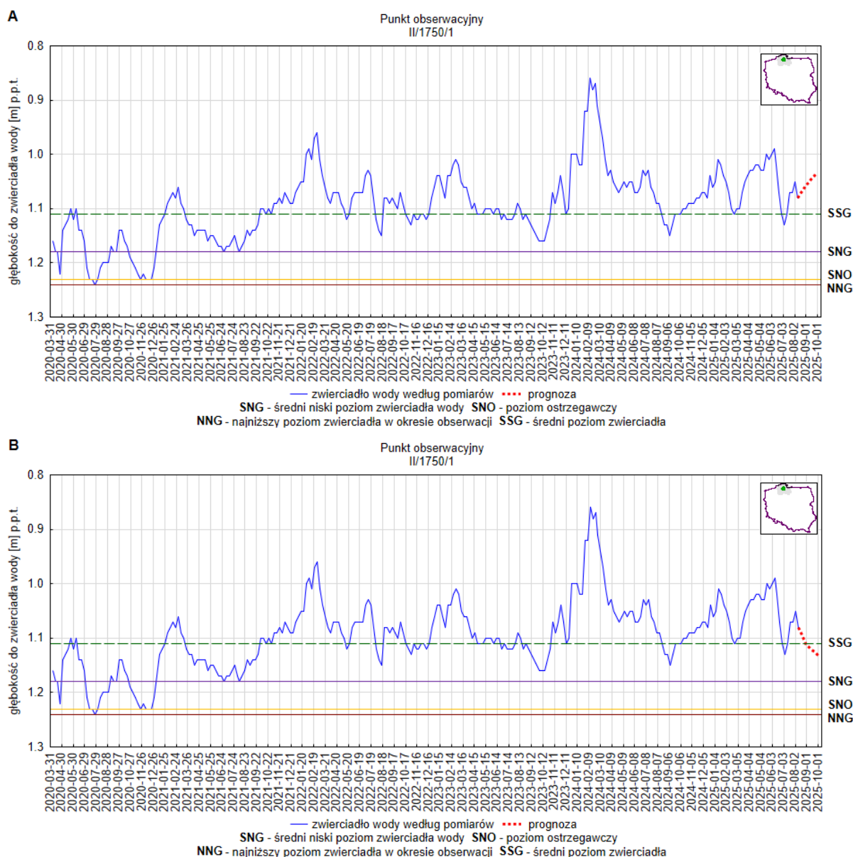
Rys. 17. Prognoza dotycząca stanu wód o zwierciadle swobodnym (gruntowych) na okres 01.09.2025 -30.09.2025 r. – stacja hydrogeologiczna nr II/1750/1 w miejscowości Borucino (woj. pomorskie). A – prognoza przy założeniu scenariusza A; B – prognoza przy założeniu scenariusza B
