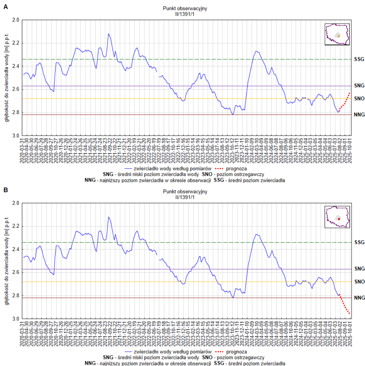
Rys. 8. Prognoza dotycząca stanu wód o zwierciadle swobodnym (gruntowych) na okres 01.09.2025 – 30.09.2025 r. – stacja hydrogeologiczna nr II/1391/1 w miejscowości Sulejów (woj. łódzkie). A – prognoza przy założeniu scenariusza A; B – prognoza przy założeniu scenariusza B
