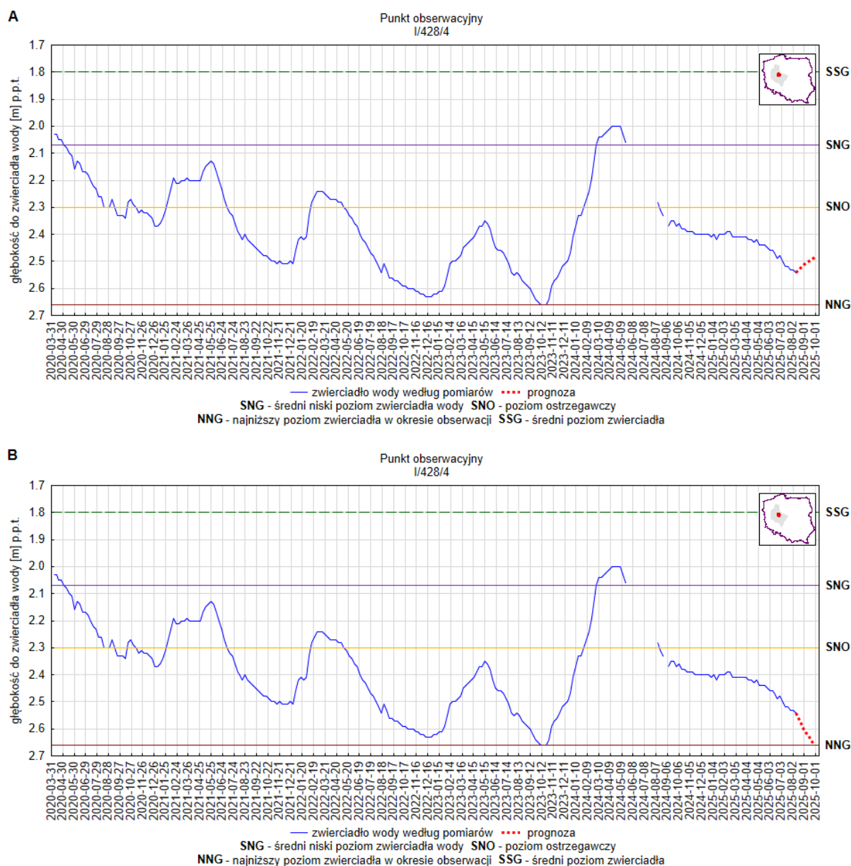
Rys. 23. Prognoza dotycząca stanu wód o zwierciadle swobodnym (gruntowych) na okres 01.09.2025 –30.09.2025 r. – stacja hydrogeologiczna nr I/428/4 w miejscowości Czachurki (woj. wielkopolskie). A – prognoza przy założeniu scenariusza A; B – prognoza przy założeniu scenariusza B
