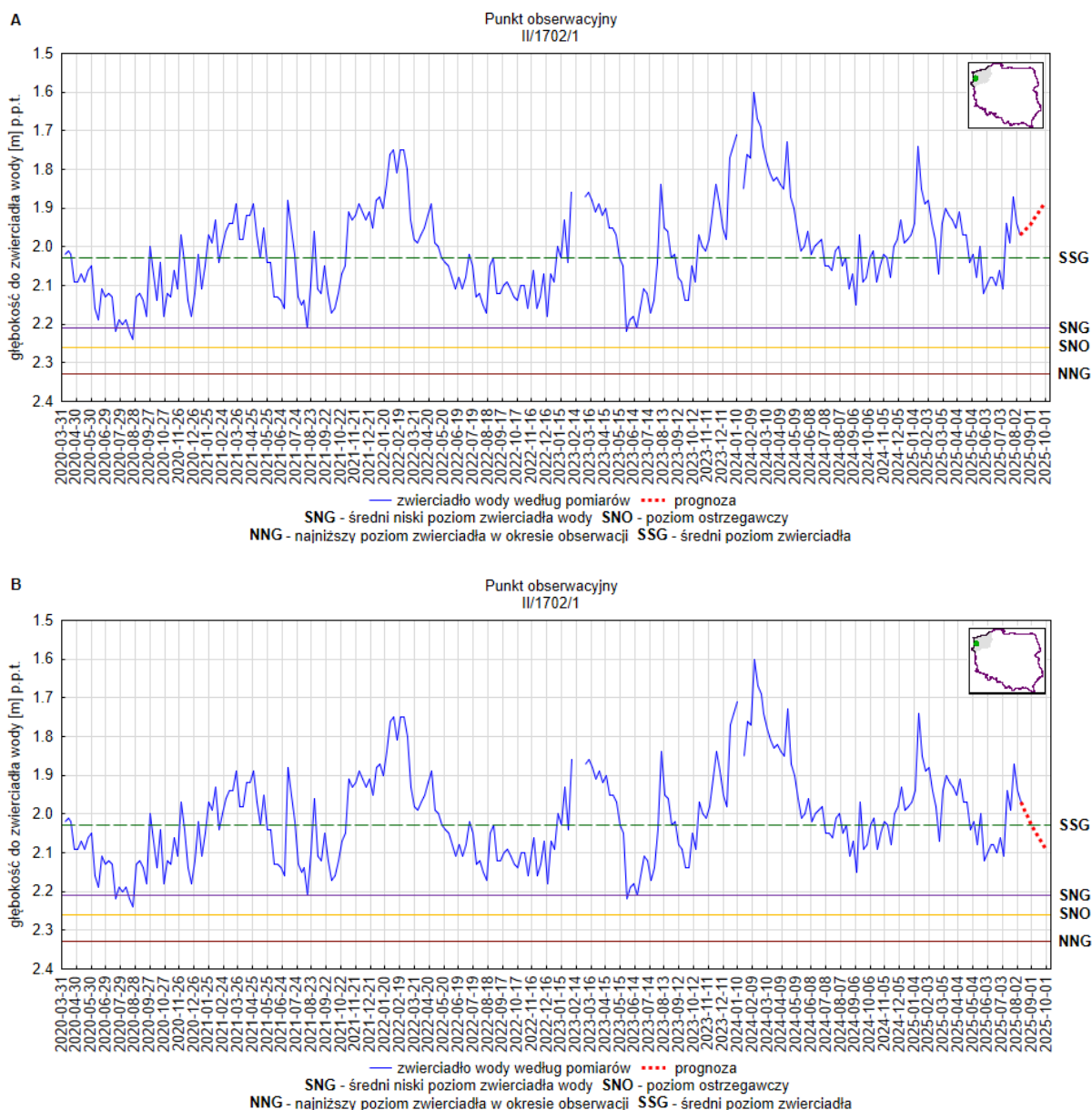
Rys. 26. Prognoza dotycząca stanu wód o zwierciadle swobodnym (gruntowych) na okres 01.09.2025 –30.09.2025 r. – stacja hydrogeologiczna nr II/1702/1 w miejscowości Szczecin (woj. zachodniopomorskie). A – prognoza przy założeniu scenariusza A; B – prognoza przy założeniu scenariusza B
