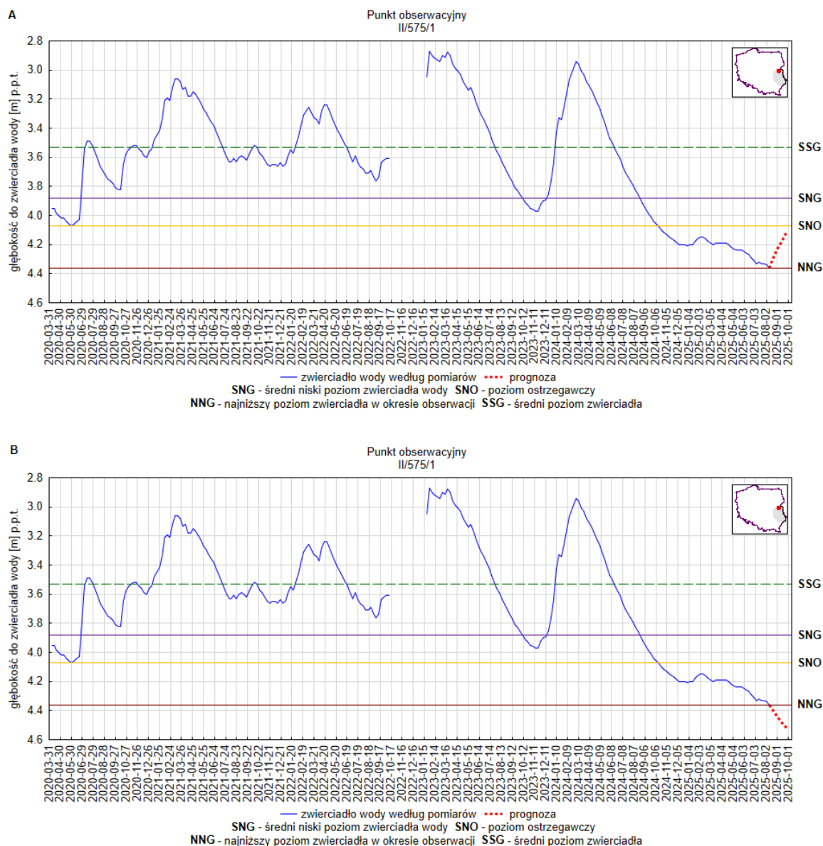
Rys. 6. Prognoza dotycząca stanu wód o zwierciadle swobodnym (gruntowych) na okres 01.09.2025 – 30.09.2025 r. – stacja hydrogeologiczna nr II/575/1 w miejscowości Manie (woj. lubelskie). A – prognoza przy założeniu scenariusza A; B – prognoza przy założeniu scenariusza B
