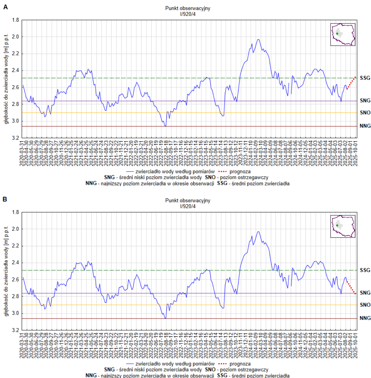
Rys. 24. Prognoza dotycząca stanu wód o zwierciadle swobodnym (gruntowych) na okres 01.09.2025 –30.09.2025 r. – stacja hydrogeologiczna nr I/920/4 w miejscowości Sepno (woj. wielkopolskie). A – prognoza przy założeniu scenariusza A; B – prognoza przy założeniu scenariusza B
