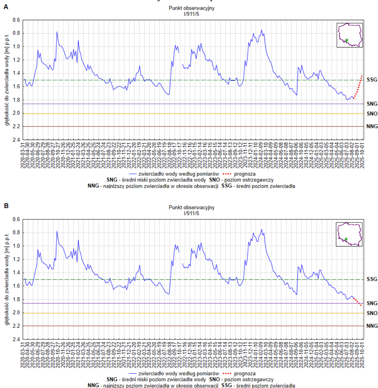
Rys. 13. Prognoza dotycząca stanu wód o zwierciadle swobodnym (gruntowych) na okres 01.09.2025 –30.09.2025 r. – stacja hydrogeologiczna nr I/911/5 w miejscowości Wrzoski (woj. opolskie). A – prognoza przy założeniu scenariusza A; B – prognoza przy założeniu scenariusza B
