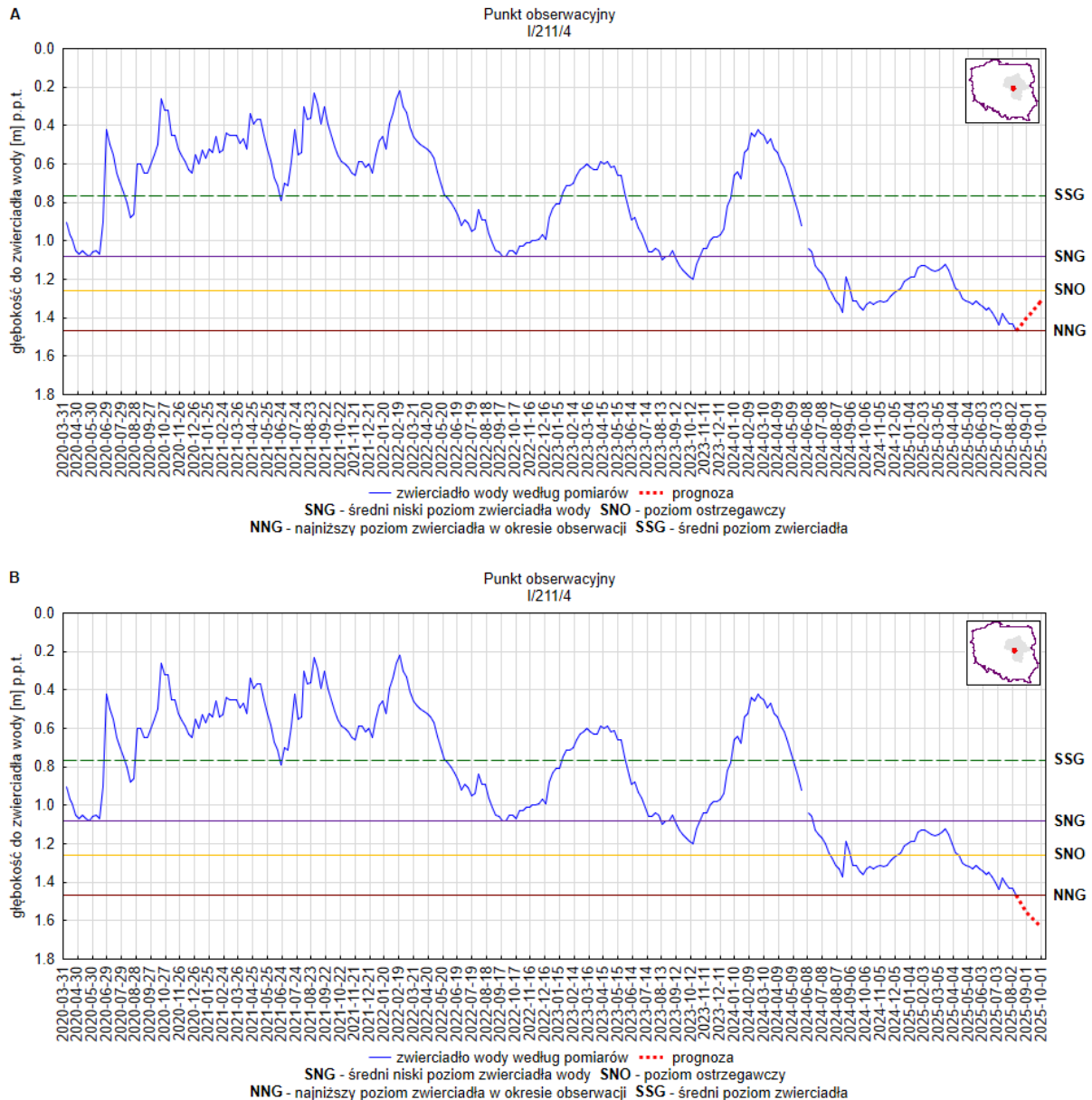
Rys. 12. Prognoza dotycząca stanu wód o zwierciadle swobodnym (gruntowych) na okres 01.09.2025 –30.09.2025 r. – stacja hydrogeologiczna nr I/211/4 w miejscowości Brwinów (woj. mazowieckie). A – prognoza przy założeniu scenariusza A; B – prognoza przy założeniu scenariusza B
