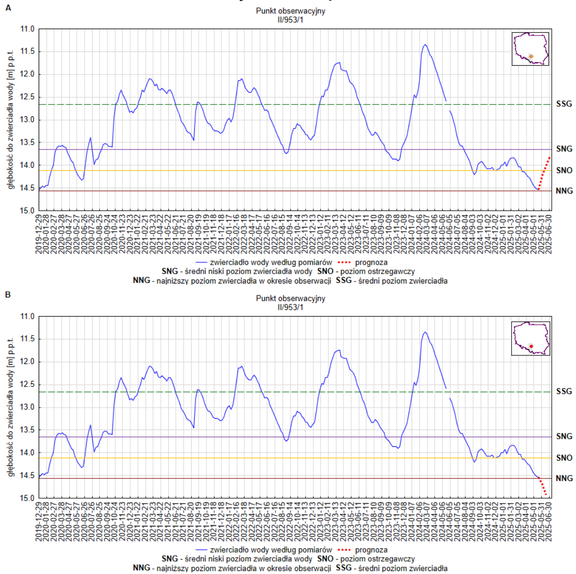
Rys. 17. Prognoza dotycząca stanu wód o zwierciadle swobodnym (gruntowych) na okres 01.06.2025 – 30.06.2025 r. – stacja hydrogeologiczna nr II/953/1 w miejscowości Żeliszawice (woj. śląskie). A – prognoza przy założeniu scenariusza A; B – prognoza przy założeniu scenariusza B
