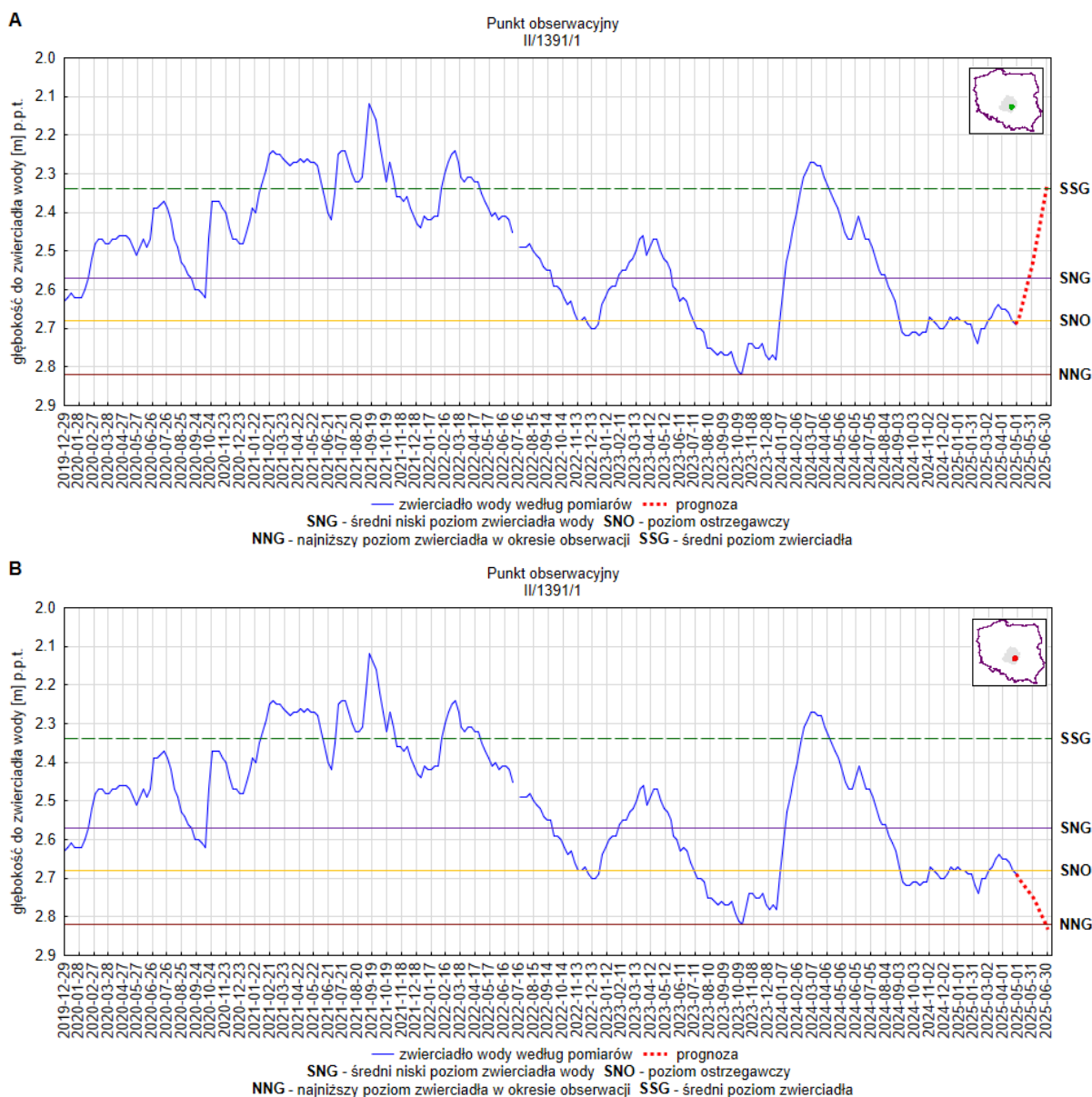
Rys. 7. Prognoza dotycząca stanu wód o zwierciadle swobodnym (gruntowych) na okres 01.06.2025 –30.06.2025 r. – stacja hydrogeologiczna nr II/1391/1 w miejscowości Sulejów (woj. łódzkie). A – prognoza przy założeniu scenariusza A; B – prognoza przy założeniu scenariusza B
