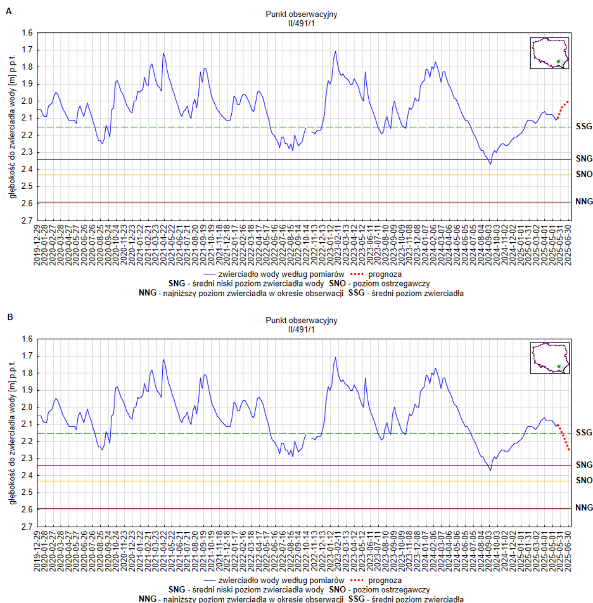
Rys. 14. Prognoza dotycząca stanu wód o zwierciadle swobodnym (gruntowych) na okres 01.06.2025 –30.06.2025 r. – stacja hydrogeologiczna nr II/491/I w miejscowości Mielec (woj. podkarpackie). A – prognoza przy założeniu scenariusza A; B – prognoza przy założeniu scenariusza B
