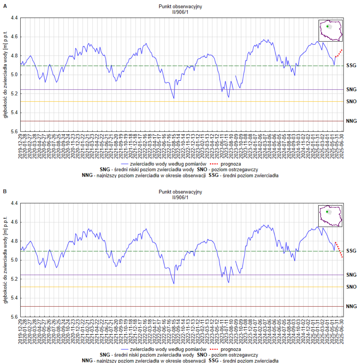
Rys. 4. Prognoza dotycząca stanu wód o zwierciadle swobodnym (gruntowych) na okres 01.06.2025 –30.06.2025 r. – stacja hydrogeologiczna nr II/906/1 w miejscowości Rozwarzyn (woj. kujawsko-pomorskie). A – prognoza przy założeniu scenariusza A; B – prognoza przy założeniu scenariusza B
