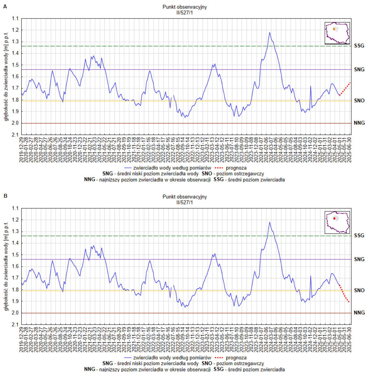
Rys. 3. Prognoza dotycząca stanu wód o zwierciadle swobodnym (gruntowych) na okres 01.06.2025 –30.06.2025 r. – stacja hydrogeologiczna nr II/527/1 w miejscowości Szubin (woj. kujawsko-pomorskie). A – prognoza przy założeniu scenariusza A; B – prognoza przy założeniu scenariusza B
