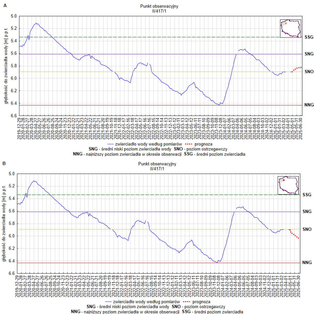
Rys. 25. Prognoza dotycząca stanu wód o zwierciadle swobodnym (gruntowych) na okres 01.06.2025 –30.06.2025 r. – stacja hydrogeologiczna nr II/417/1 w miejscowości Turowo (woj. zachodniopomorskie). A – prognoza przy założeniu scenariusza A; B – prognoza przy założeniu scenariusza B
