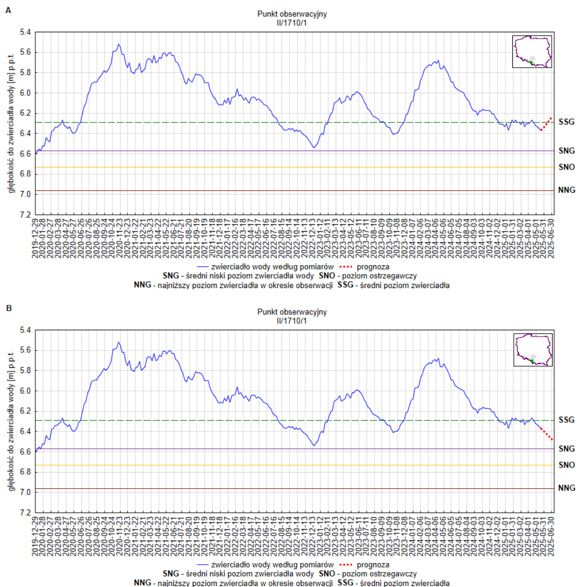
Rys. 18. Prognoza dotycząca stanu wód o zwierciadle swobodnym (gruntowych) na okres 01.06.2025 – 30.06.2025 r. – stacja hydrogeologiczna nr II/1710/1 w miejscowości Gołysz (woj. śląskie). A – prognoza przy założeniu scenariusza A; B – prognoza przy założeniu scenariusza B
