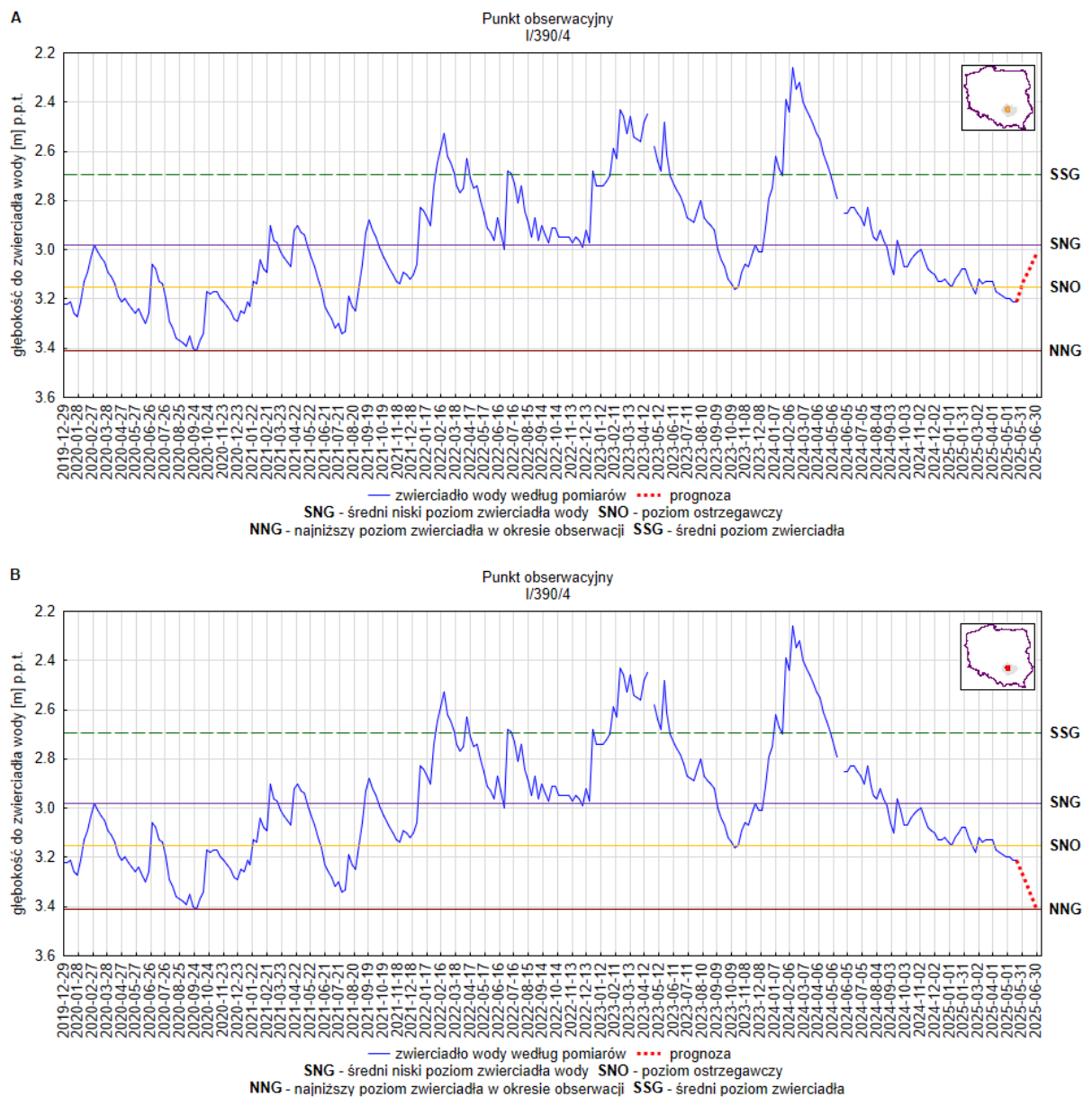
Rys. 19. Prognoza dotycząca stanu wód o zwierciadle swobodnym (gruntowych) na okres 01.06.2025 –30.06.2025 r. – stacja hydrogeologiczna nr I/390/4 w miejscowości Nałęczów (woj. świętokrzyskie). A – prognoza przy założeniu scenariusza A; B – prognoza przy założeniu scenariusza B
