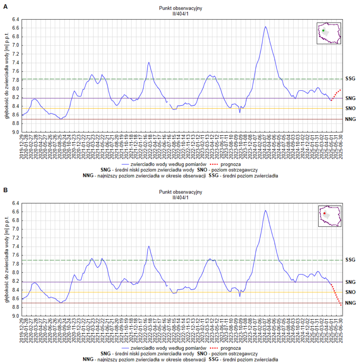
Rys. 23. Prognoza dotycząca stanu wód o zwierciadle swobodnym (gruntowych) na okres 01.06.2025 –30.06.2025 r. – stacja hydrogeologiczna nr II/404/1 w miejscowości Obrzycko (woj. wielkopolskie). A – prognoza przy założeniu scenariusza A; B – prognoza przy założeniu scenariusza B
