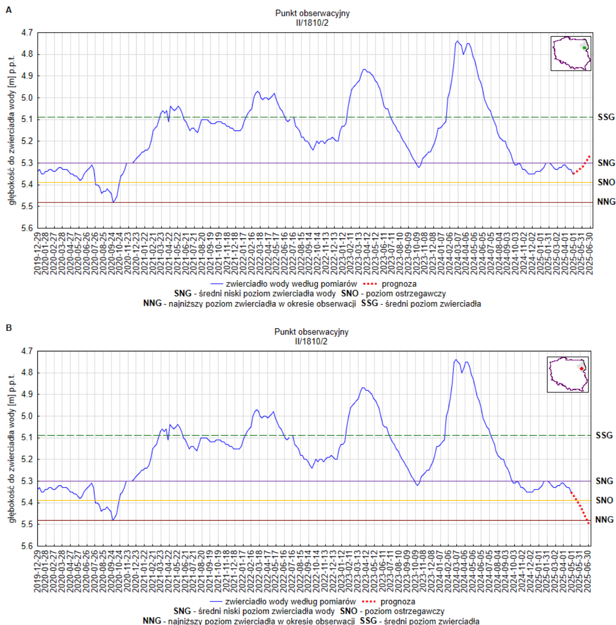
Rys. 15. Prognoza dotycząca stanu wód o zwierciadle swobodnym (gruntowych) na okres 01.06.2025 –30.06.2025 r.- stacja hydrogeologiczna nr II/1810/2 w miejscowości Liza Stara (woj. podlaskie). A – prognoza przy założeniu scenariusza A; B – prognoza przy założeniu scenariusza B
