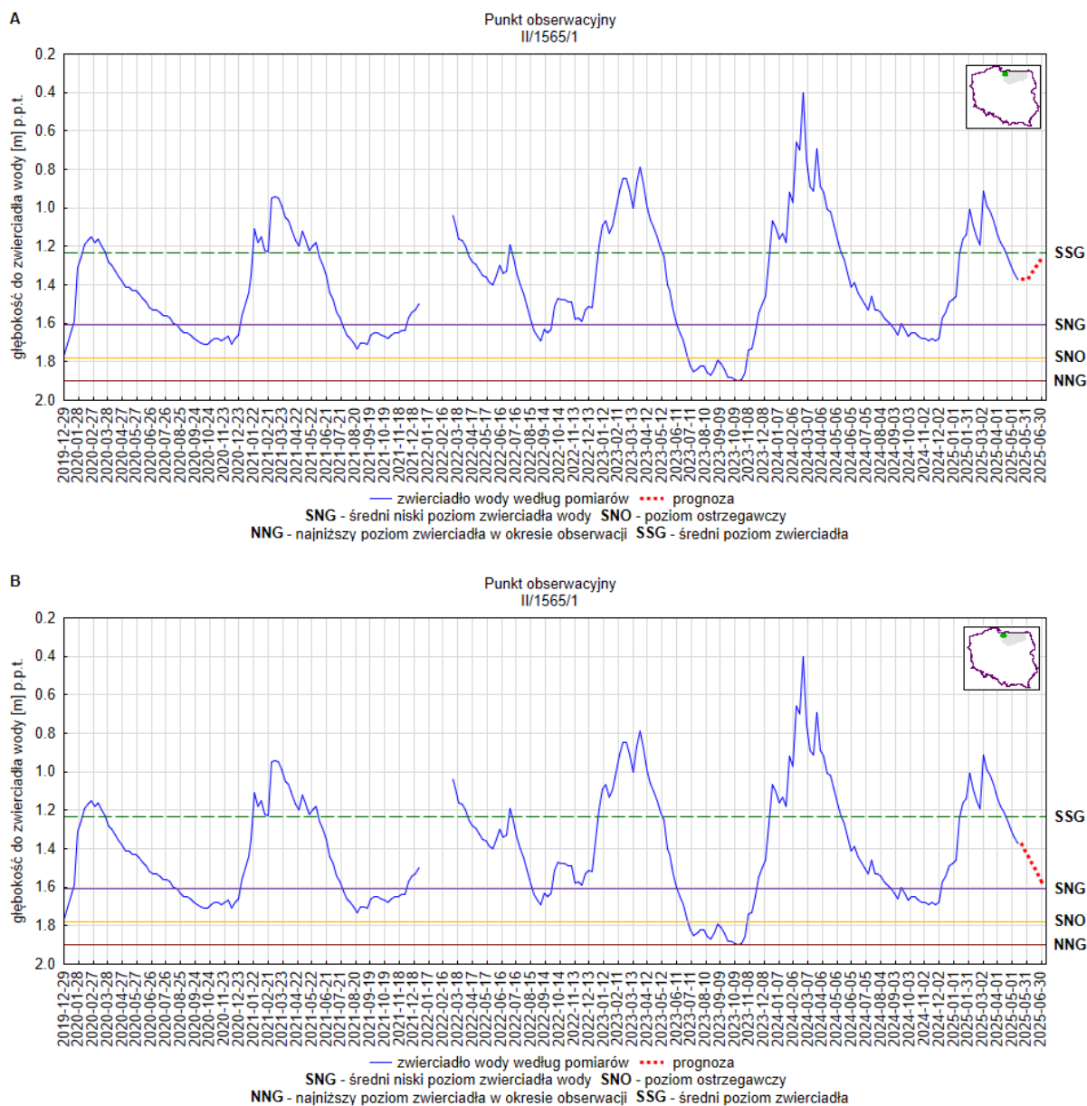
Rys. 22. Prognoza dotycząca stanu wód o zwierciadle swobodnym (gruntowych) na okres 01.06.2025 –30.06.2025 r. – stacja hydrogeologiczna nr II/1565/1 w miejscowości Karczowiska Górne (woj. warmińsko-mazurskie). A – prognoza przy założeniu scenariusza A; B – prognoza przy założeniu scenariusza B
