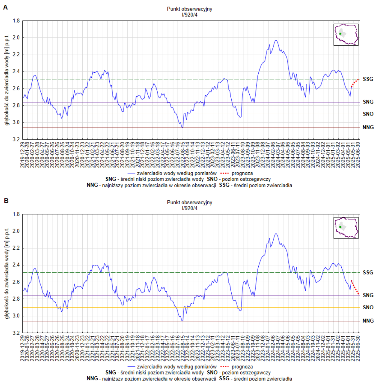
Rys. 24. Prognoza dotycząca stanu wód o zwierciadle swobodnym (gruntowych) na okres 01.06.2025 –30.06.2025 r. – stacja hydrogeologiczna nr I/920/4 w miejscowości Sepno (woj. wielkopolskie). A – prognoza przy założeniu scenariusza A; B – prognoza przy założeniu scenariusza B
