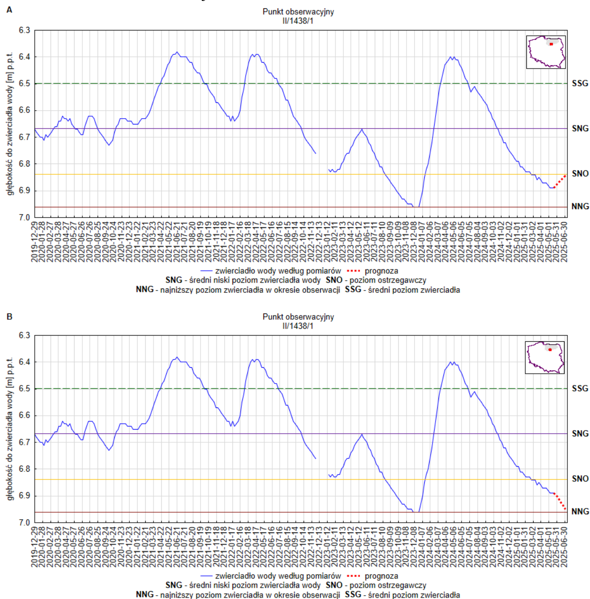
Rys. 21. Prognoza dotycząca stanu wód o zwierciadle swobodnym (gruntowych) na okres 01.06.2025 –30.06.2025 r. – stacja hydrogeologiczna nr II/1438/1 w miejscowości Muszaki (woj. warmińsko-mazurskie). A – prognoza przy założeniu scenariusza A; B – prognoza przy założeniu scenariusza B
