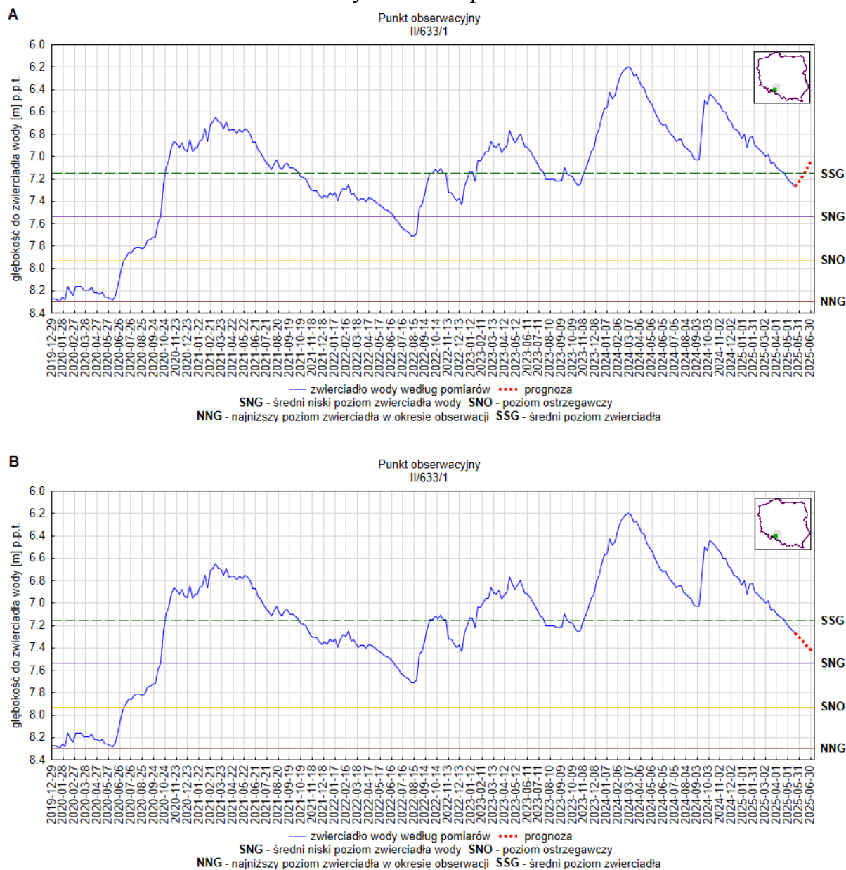
Rys. 12. Prognoza dotycząca stanu wód o zwierciadle swobodnym (gruntowych) na okres 01.06.2025 –30.06.2025 r. – stacja hydrogeologiczna nr II/633/1 w miejscowości Łącznik (woj. opolskie). A – prognoza przy założeniu scenariusza A; B – prognoza przy założeniu scenariusza B
