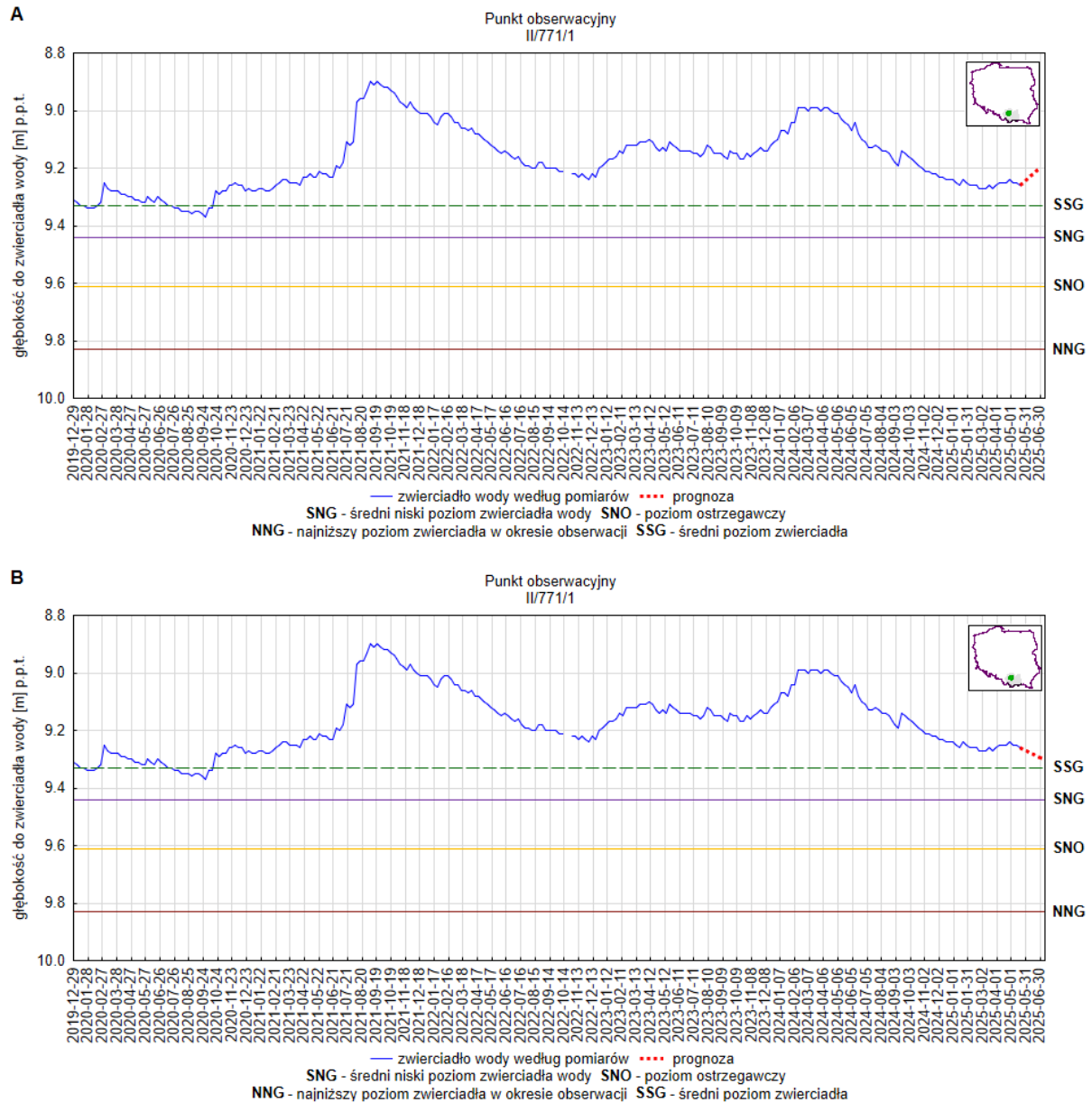
Rys. 9. Prognoza dotycząca stanu wód o zwierciadle swobodnym (gruntowych) na okres 01.06.2025 – 30.06.2025 r. – stacja hydrogeologiczna nr II/771/1 w miejscowości Kraków (woj. małopolskie). A – prognoza przy założeniu scenariusza A; B – prognoza przy założeniu scenariusza B
