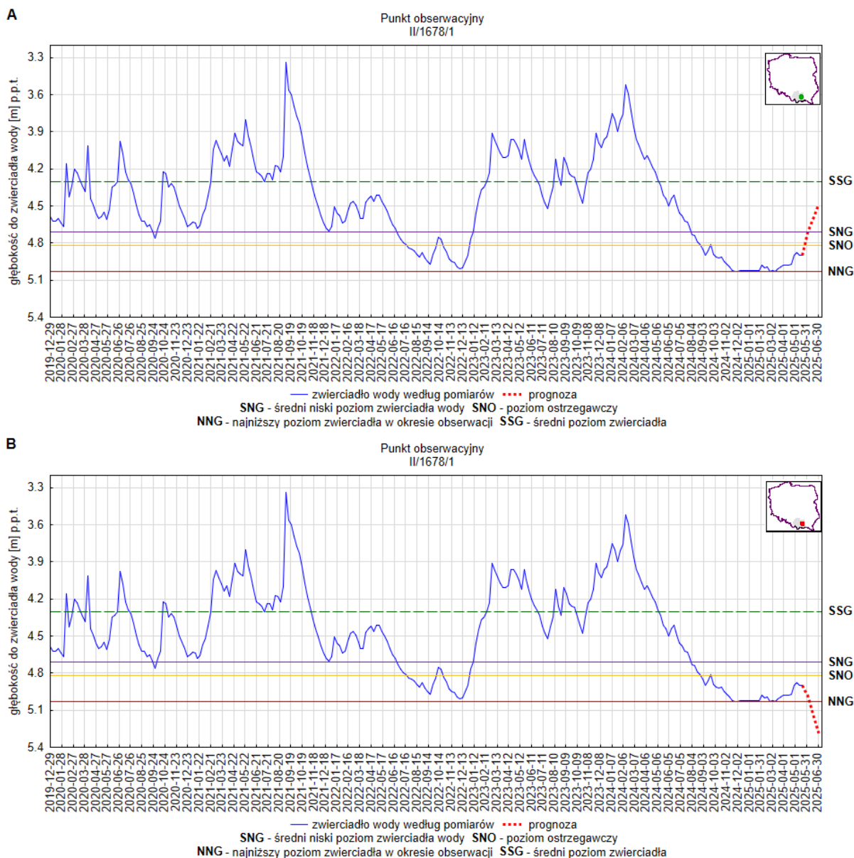
Rys. 8. Prognoza dotycząca stanu wód o zwierciadle swobodnym (gruntowych) na okres 01.06.2025 – 30.06.2025 r. – stacja hydrogeologiczna nr II/1678/1 w miejscowości Zakliczyn (woj. małopolskie). A – prognoza przy założeniu scenariusza A; B – prognoza przy założeniu scenariusza B
