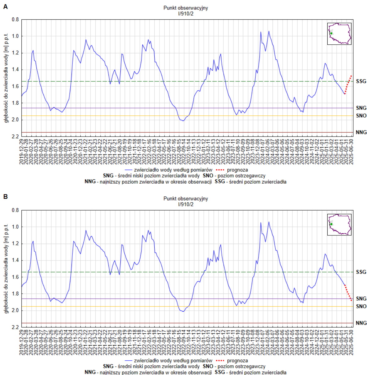
Rys. 6. Prognoza dotycząca stanu wód o zwierciadle swobodnym (gruntowych) na okres 01.06.2025 – 30.06.2025 r. – stacja hydrogeologiczna nr I/910/2 w miejscowości Wysokie (woj. lubuskie) A – prognoza przy założeniu scenariusza A; B – prognoza przy założeniu scenariusza B
