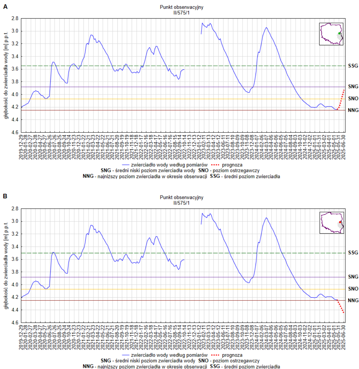
Rys. 5. Prognoza dotycząca stanu wód o zwierciadle swobodnym (gruntowych) na okres 01.06.2025 –30.06.2025 r. – stacja hydrogeologiczna nr II/575/1 w miejscowości Manie (woj. lubelskie). A – prognoza przy założeniu scenariusza A; B – prognoza przy założeniu scenariusza B
