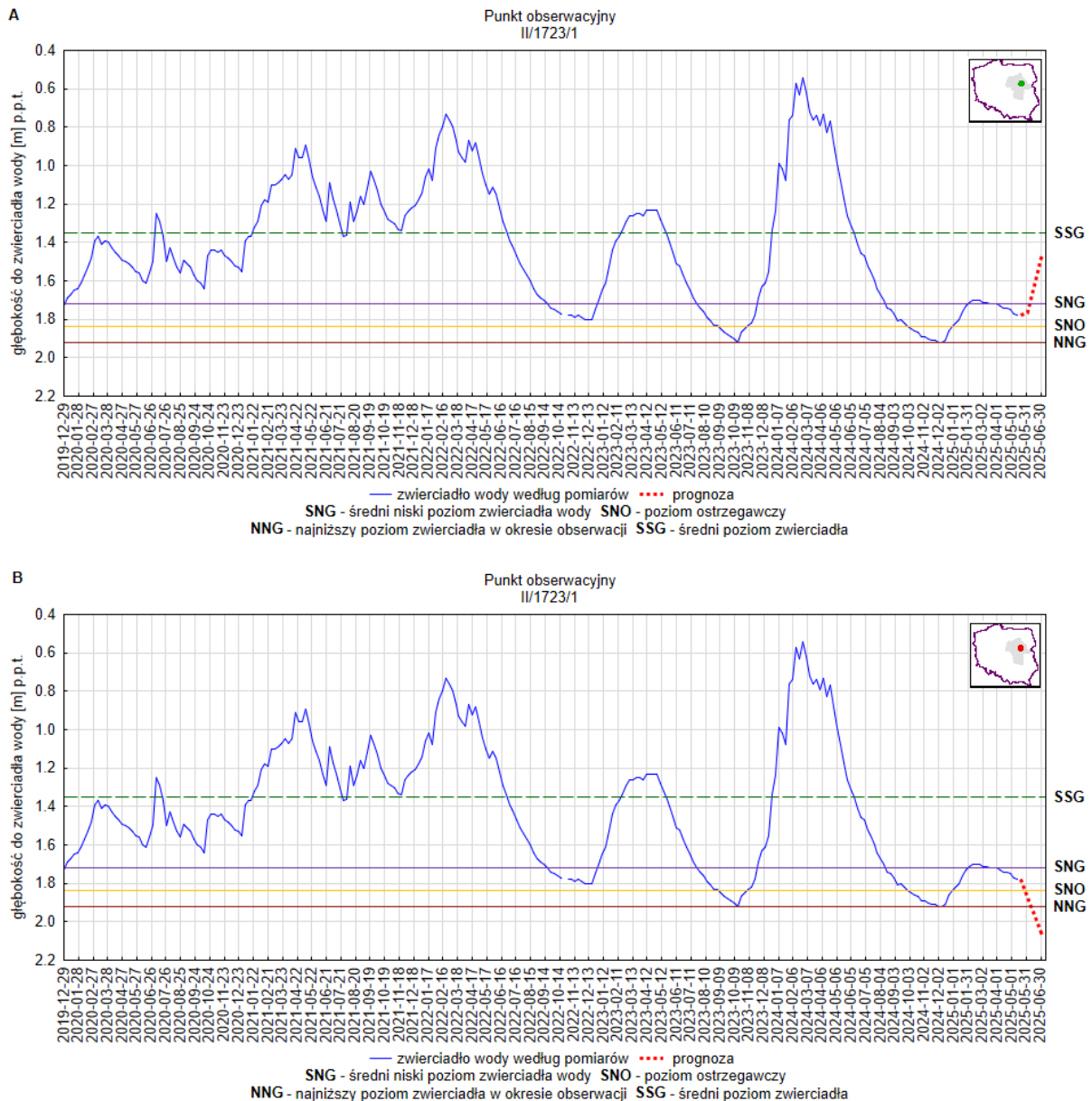
Rys. 10. Prognoza dotycząca stanu wód o zwierciadle swobodnym (gruntowych) na okres 01.06.2025 – 30.06.2025 r. – stacja hydrogeologiczna nr II/1723/1 w miejscowości Kaliska (woj. mazowieckie). A – prognoza przy założeniu scenariusza A; B – prognoza przy założeniu scenariusza B
