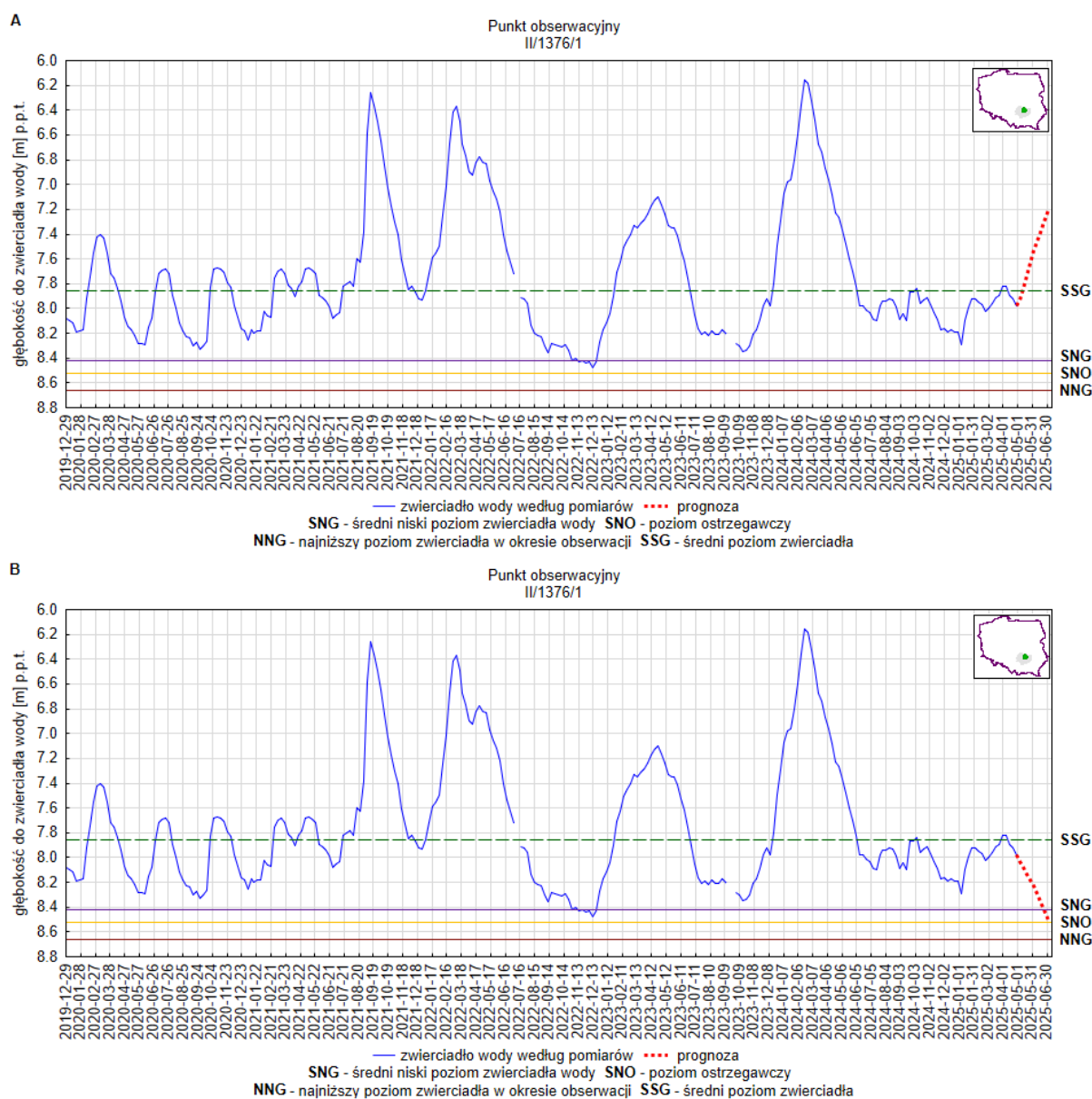
Rys. 20. Prognoza dotycząca stanu wód o zwierciadle swobodnym (gruntowych) na okres 01.06.2025 –30.06.2025 r. – stacja hydrogeologiczna nr II/1376/1 w miejscowości Bodzentyn (woj. świętokrzyskie). A – prognoza przy założeniu scenariusza A; B – prognoza przy założeniu scenariusza B
