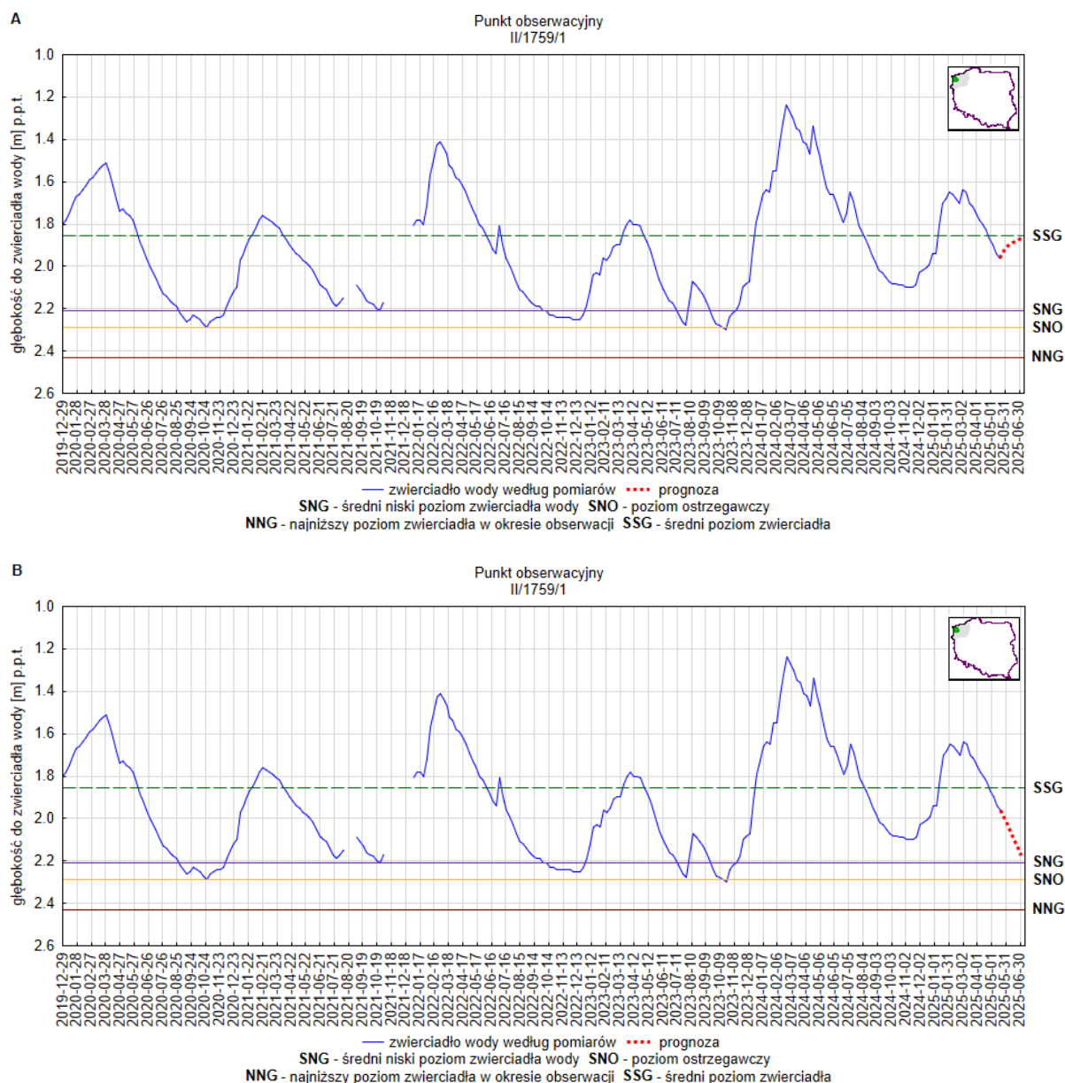
Rys. 26. Prognoza dotycząca stanu wód o zwierciadle swobodnym (gruntowych) na okres 01.06.2025 – 30.06.2025 r. – stacja hydrogeologiczna nr II/1759/1 w miejscowości Krępsko (woj. zachodniopomorskie). A – prognoza przy założeniu scenariusza A; B – prognoza przy założeniu scenariusza B
