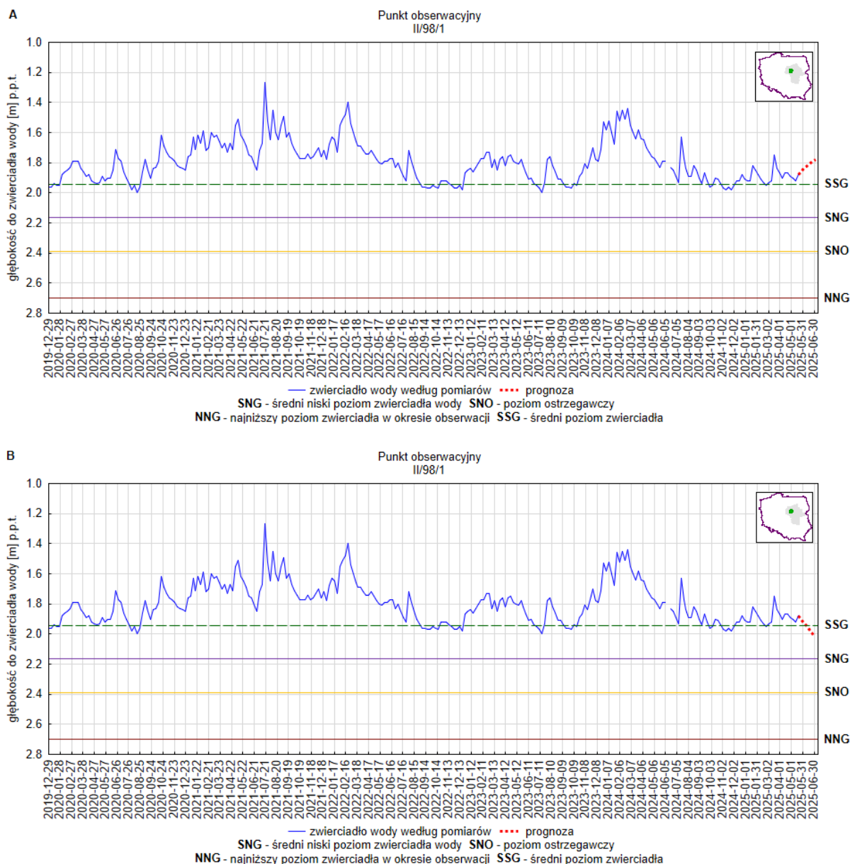
Rys. 11. Prognoza dotycząca stanu wód o zwierciadle swobodnym (gruntowych) na okres 01.06.2025 –30.06.2025 r. – stacja hydrogeologiczna nr II/98/1 w miejscowości Płońsk (woj. mazowieckie). A – prognoza przy założeniu scenariusza A; B – prognoza przy założeniu scenariusza B
