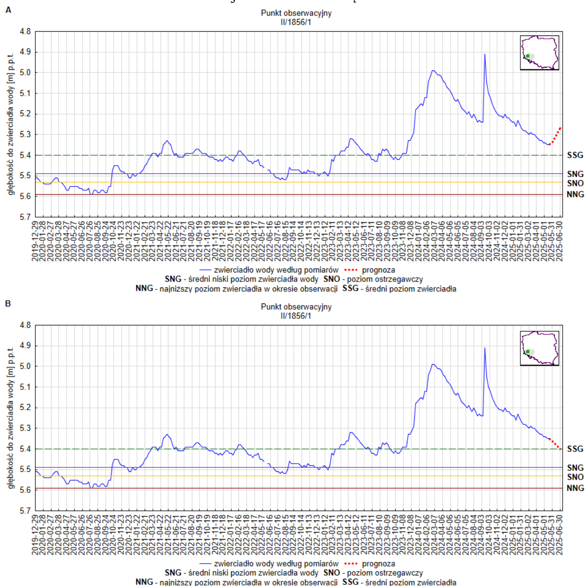
Rys. 2. Prognoza dotycząca stanu wód o zwierciadle swobodnym (gruntowych) na okres 01.06.2025 – 30.06.2025 r. – stacja hydrogeologiczna nr II/1856/1 w miejscowości Goliszów (woj. dolnośląskie). A – prognoza przy założeniu scenariusza A; B – prognoza przy założeniu scenariusza B
