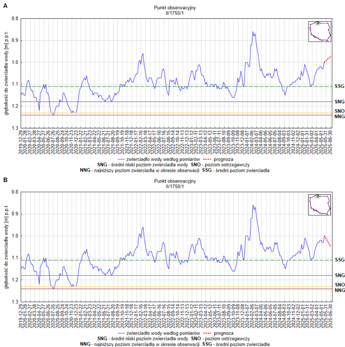
Rys. 16. Prognoza dotycząca stanu wód o zwierciadle swobodnym (gruntowych) na okres 01.06.2025 -30.06.2025 r. – stacja hydrogeologiczna nr II/1750/1 w miejscowości Borucino (woj. pomorskie). A – prognoza przy założeniu scenariusza A; B – prognoza przy założeniu scenariusza B
