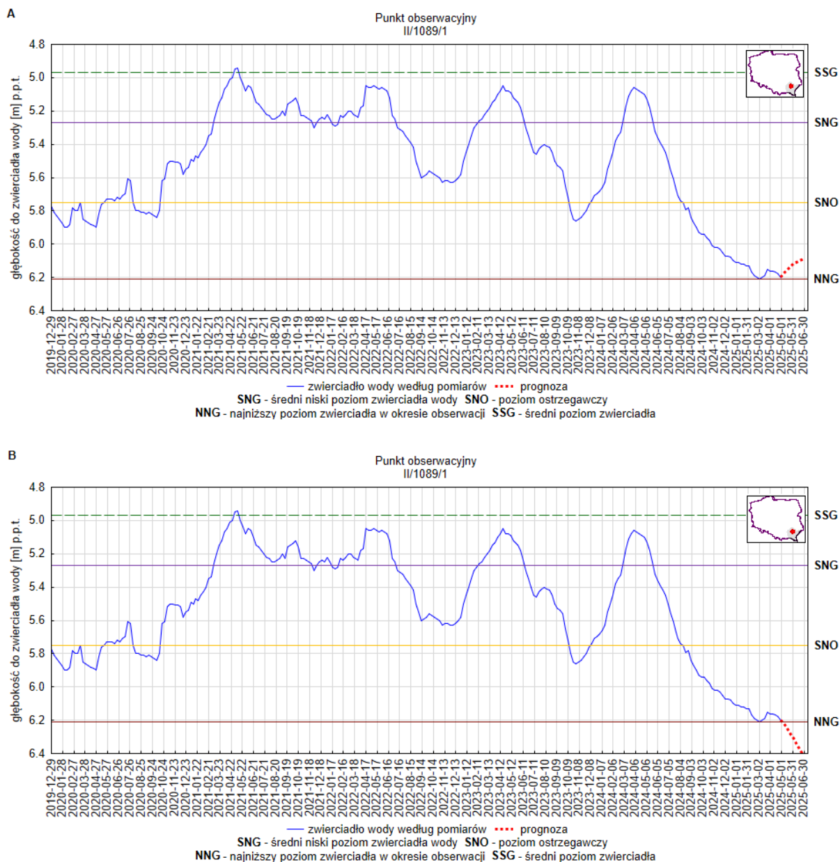
Rys. 13. Prognoza dotycząca stanu wód o zwierciadle swobodnym (gruntowych) na okres 01.06.2025 – 30.06.2025 r. – stacja hydrogeologiczna nr II/1089/1 w miejscowości Turza (woj. podkarpackie). A – prognoza przy założeniu scenariusza A; B – prognoza przy założeniu scenariusza B
